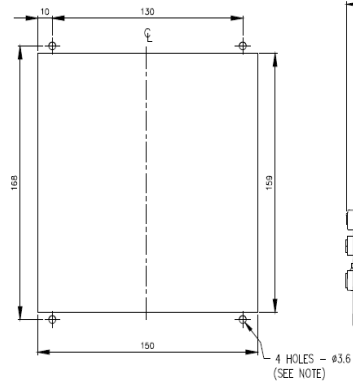
PANEL CUT-OUT/SCHALTAFELAUSSCHNITT
