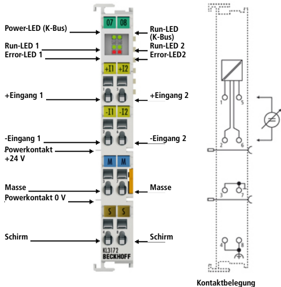
Kontaktbelegung
