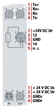
Steckerbelegung
