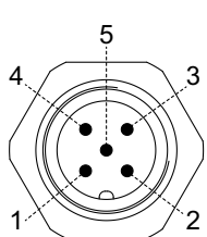
Stecker M12 (Stift, A 1) ) 5-polig, A-codiert
