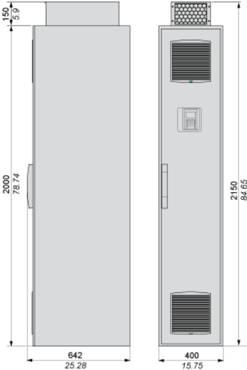
Rechtsseitige Ansicht und Vorderansicht
