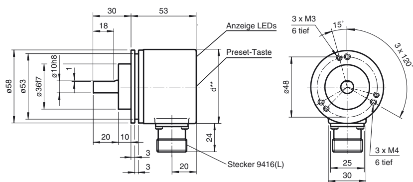
Klemmflansch
