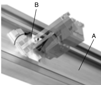
Montage des Haltewinkels am Trägerprofil
