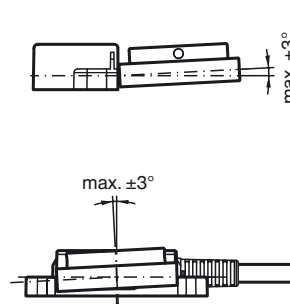
Winkelversatz
