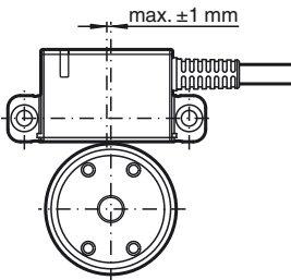
Achsversatz
