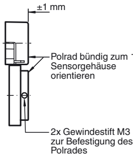
Einbau
