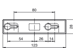
Montagemaße für Drehbügel
