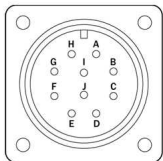
10 Pin MS3102R
