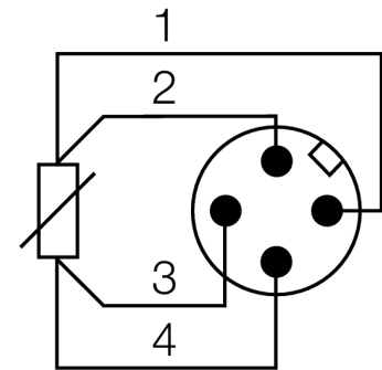
接线图
