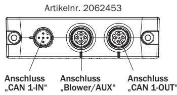
Anschluss „Blower/AUX“, V_S, I_{out\ max} = 4\ A
