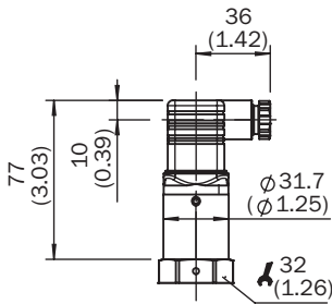
Rysunek wymiarowy: obudowa
