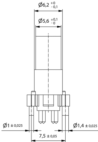
Габаритный чертёж
